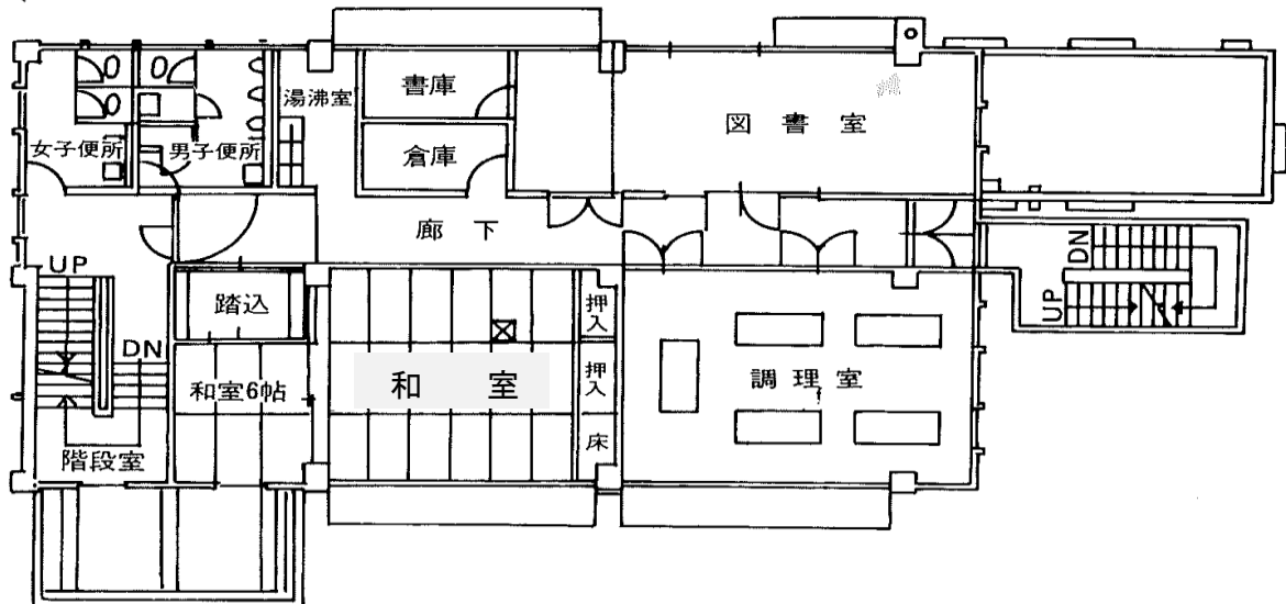
(3階平面)
