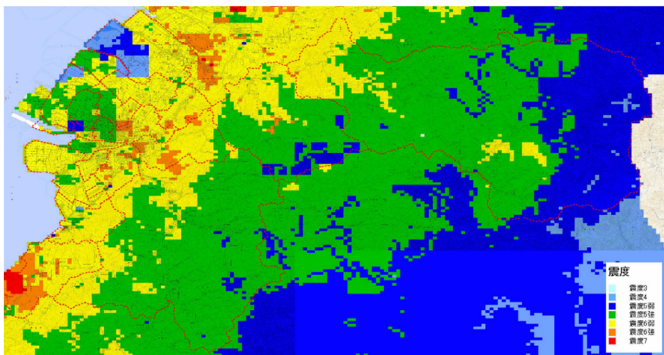
図 1.1.2 布田川・日奈久断層帯(中部・南西部連動)を震源とした地震における震度想定 (八代市建築物耐震促進計画資料編より)
