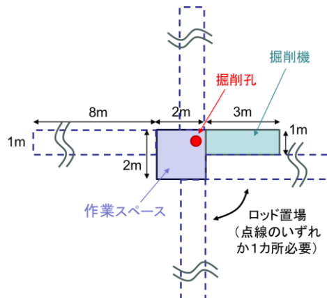
井戸掘削に必要な作業スペース(平面図)
