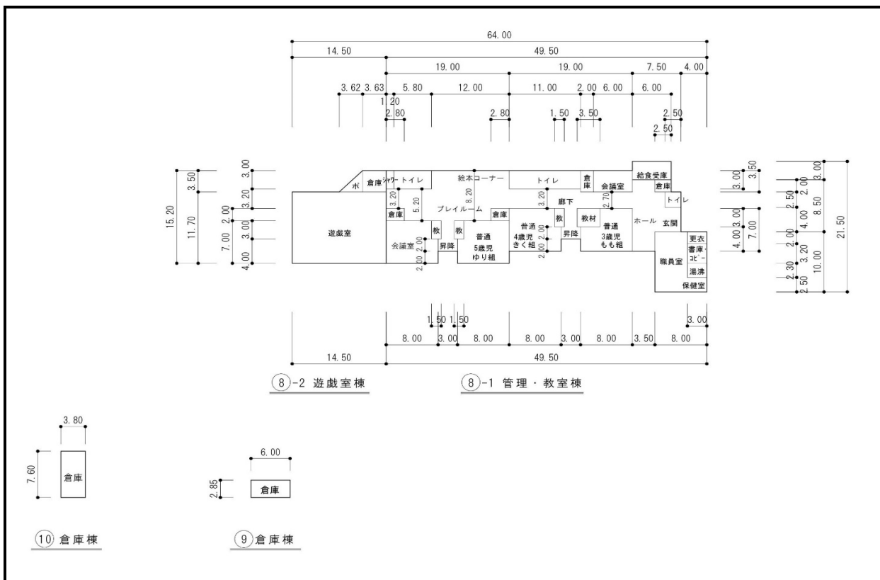
(4) 平面図 (建物が複数ある場合は、主要なもの)
