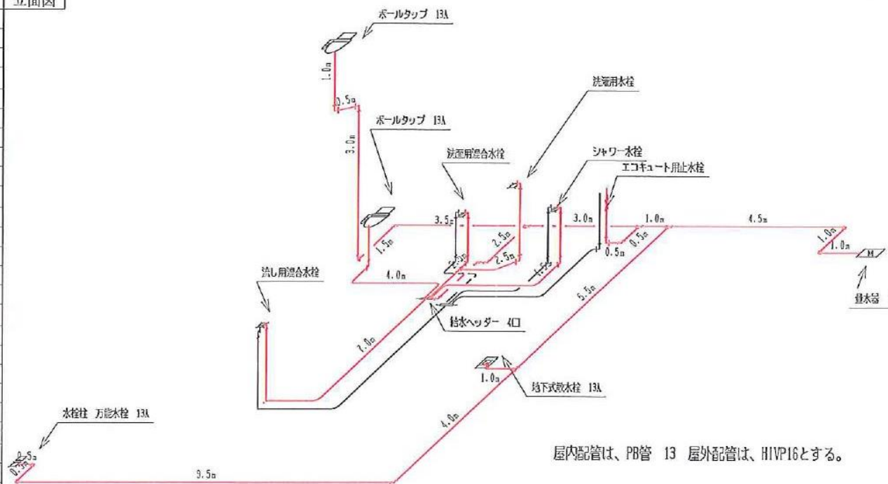
立面図
