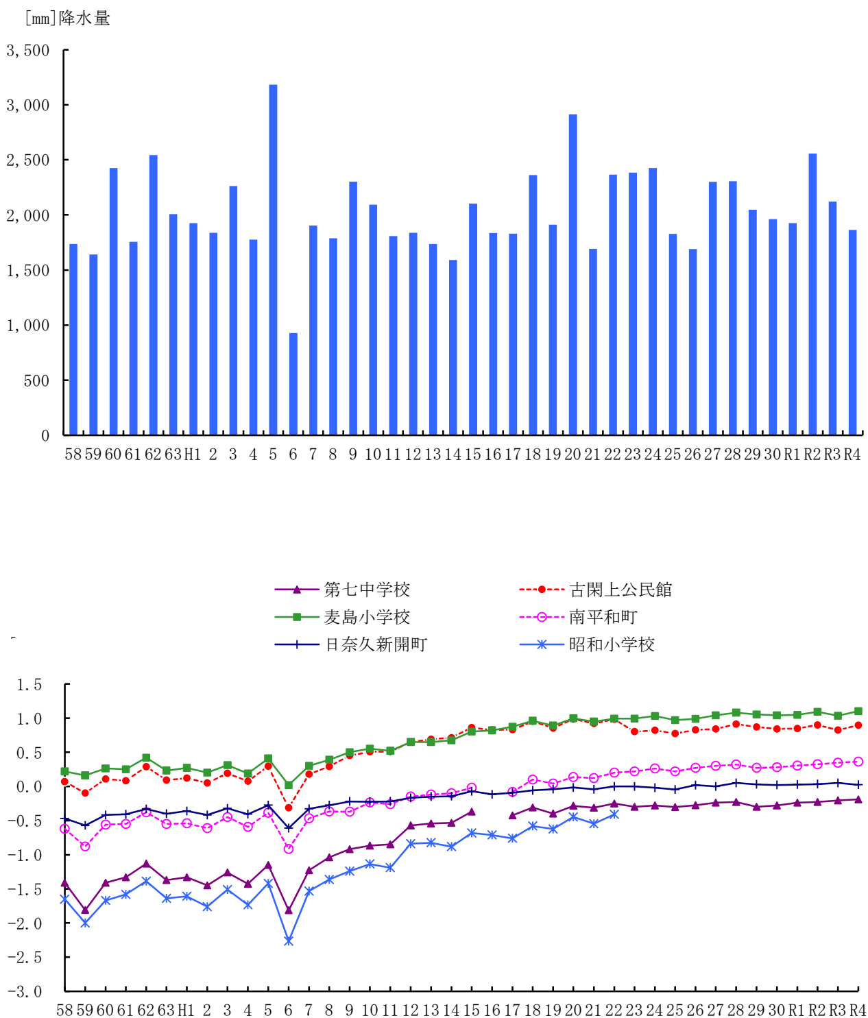
図－2 降水量と年平均水位の経年変化
