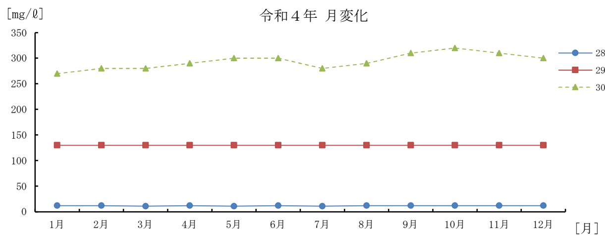
図－9 地域別塩化物イオン濃度の幾何平均の修正移動平均値の推移
