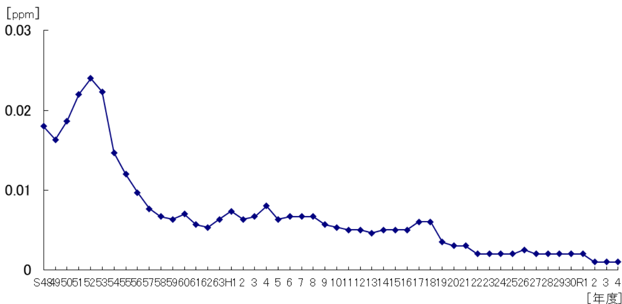
図－2 二酸化硫黄の自動測定結果による経年変化
