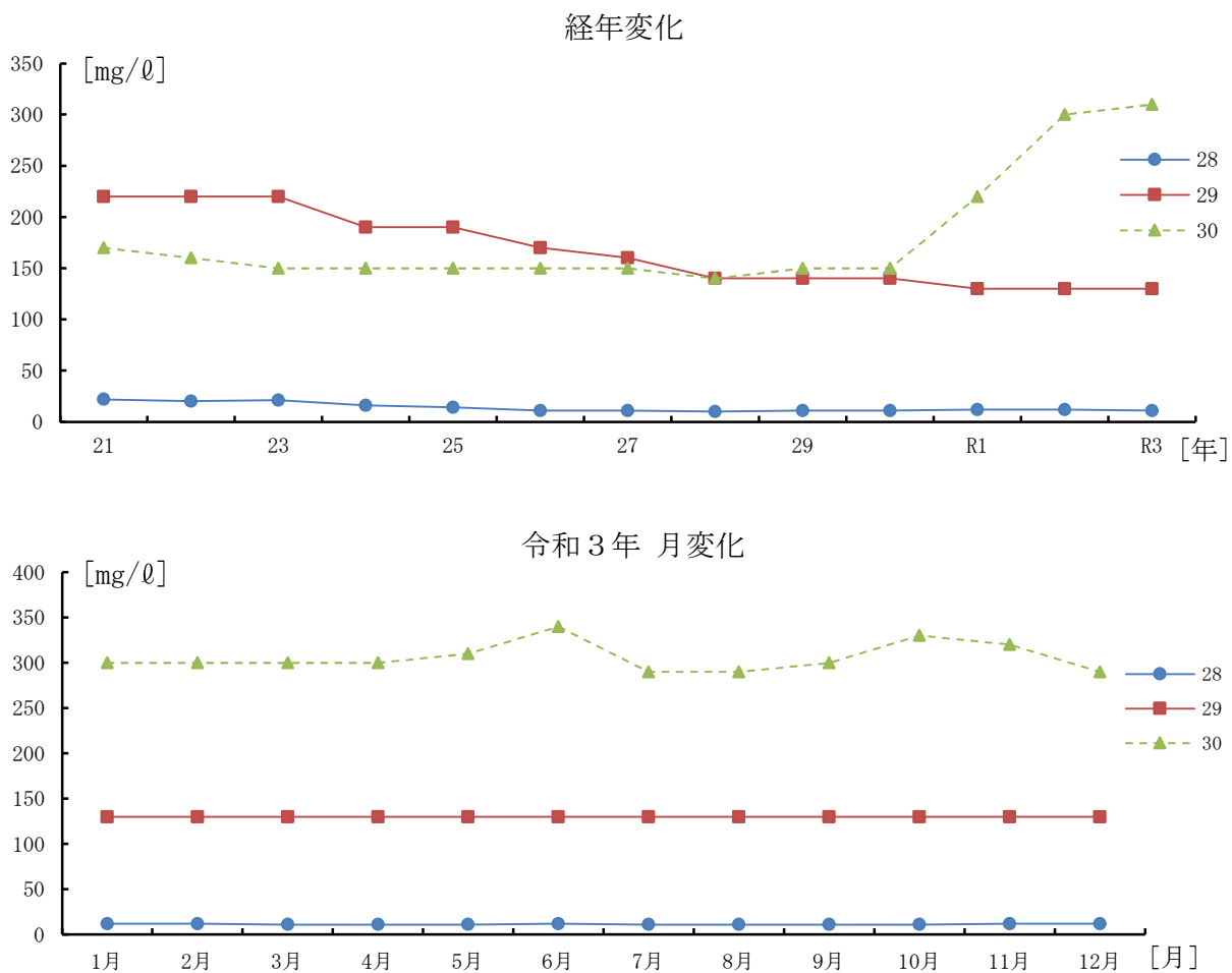
図－8 鏡地区
