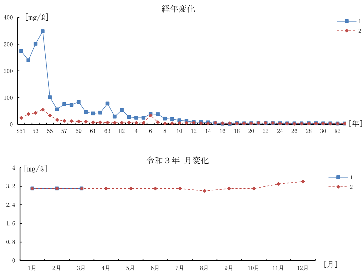
図－3 水島地区
