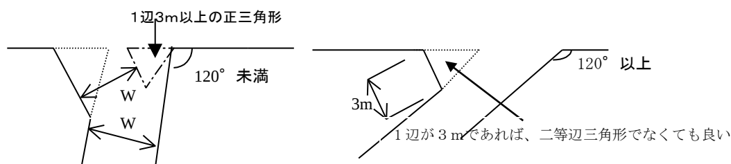
図4-3-2 片隅切り
