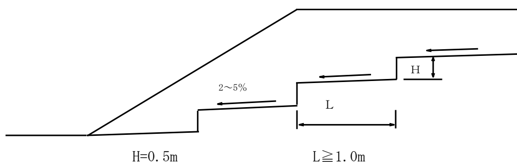
図4-9-2 段切り
