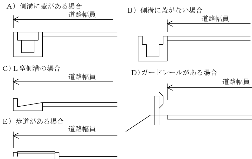
図4-3-1 道路幅員
