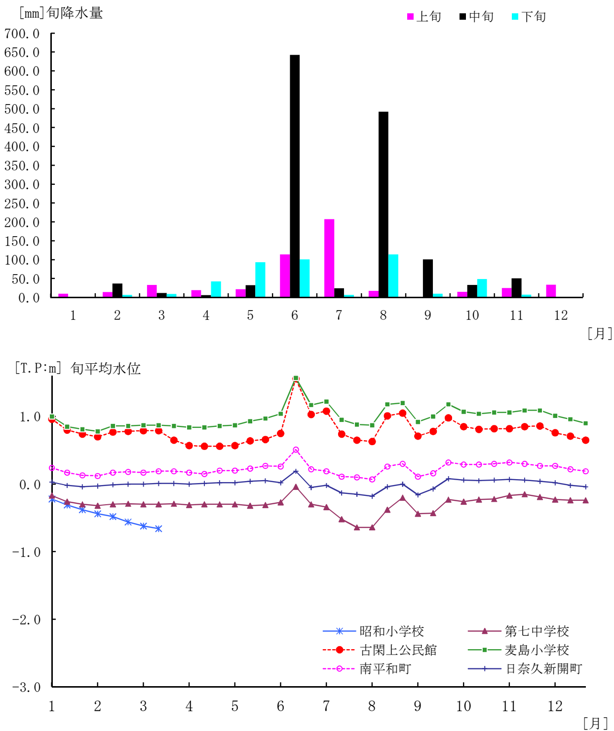
図－3 平成23年旬降水量と旬平均水位の変動
