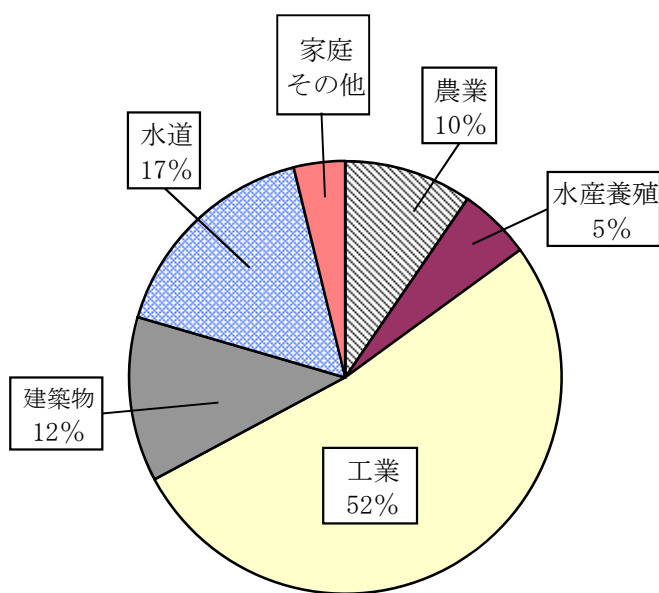
図－2 平成22年度地下水採取量内訳
