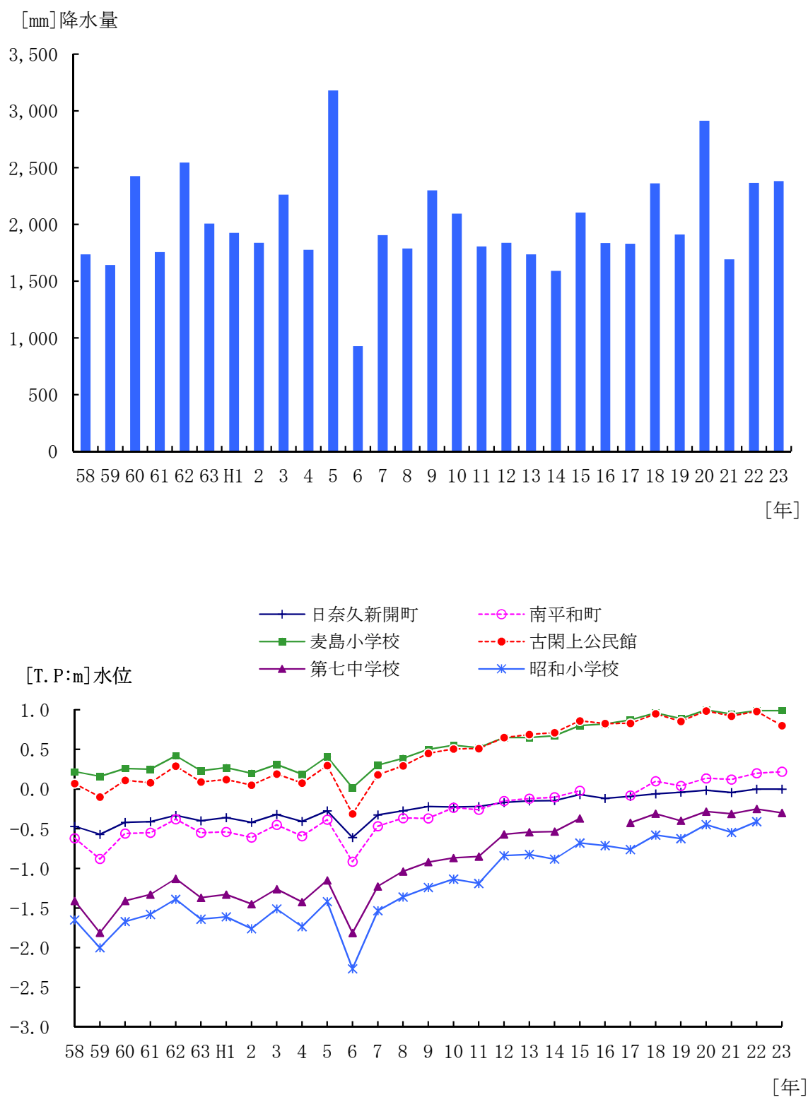
図－２ 降水量と年平均水位の経年変化
