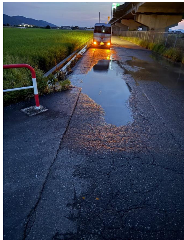
高速側道部 300mm 鑄鉄管
