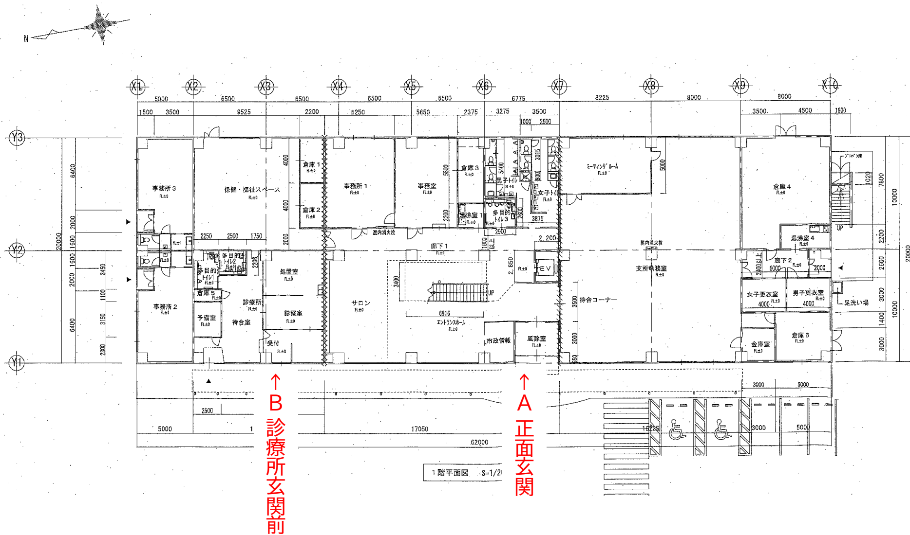
坂本支所1階平面図
