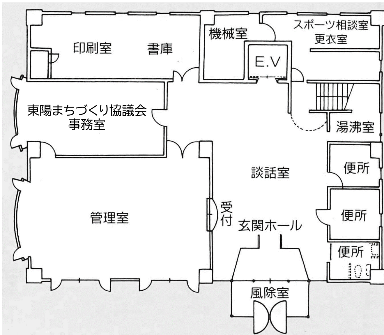
東陽コミュニティセンター1階平面図
