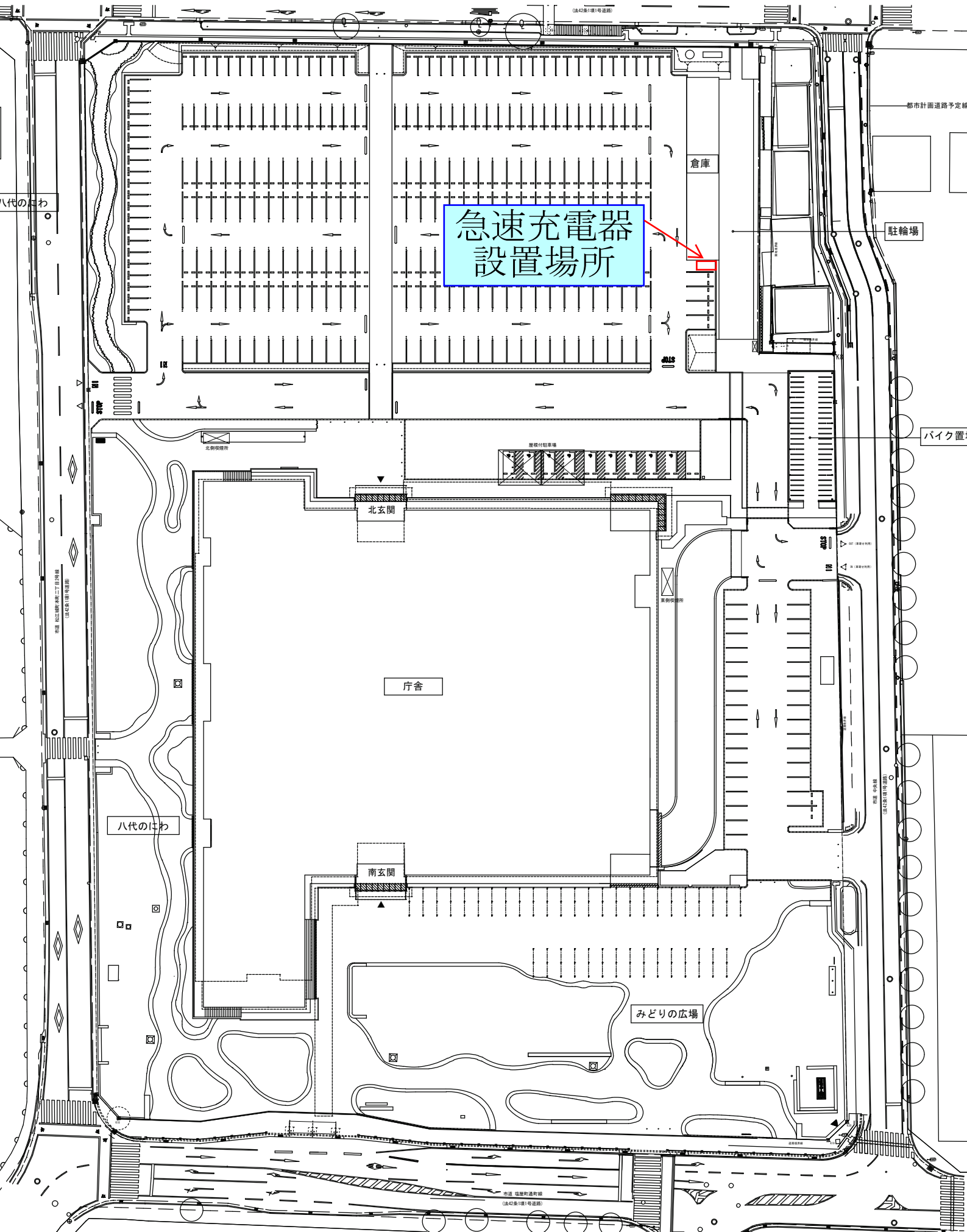
八代市役所 全体配置図
