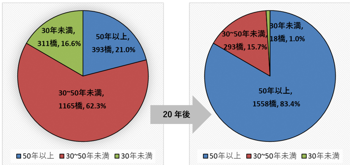
図 1.1.4 架設後 50 年超橋梁の推移
