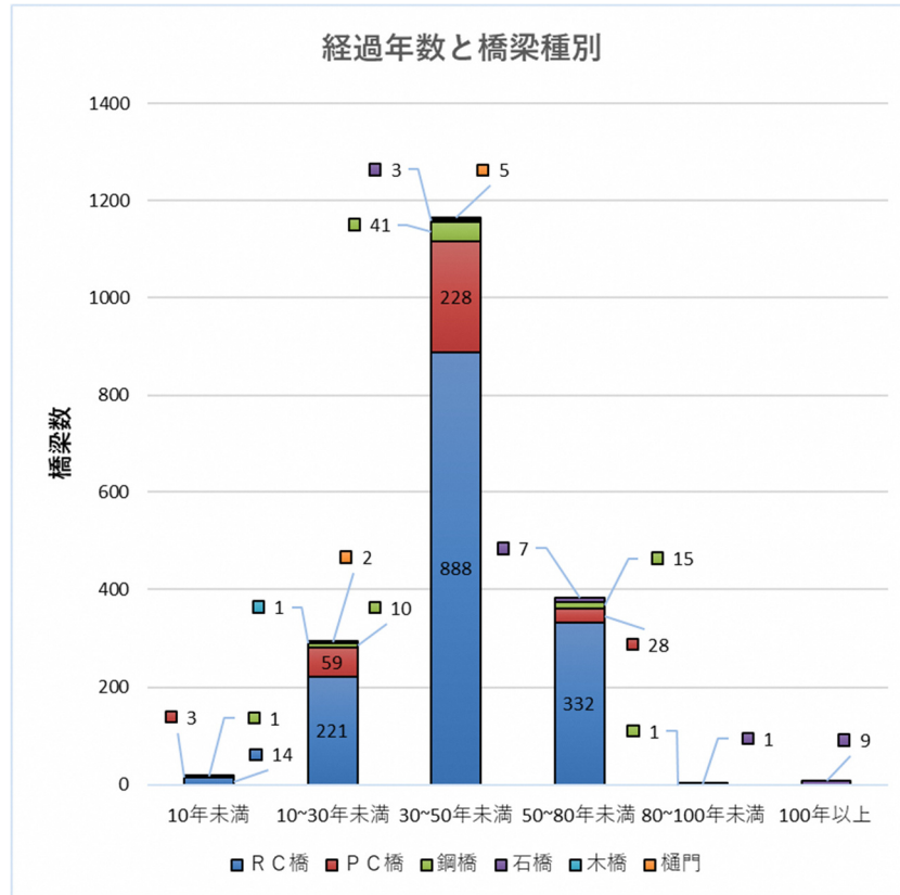
図 1.1.7 経過年数と橋梁種別
