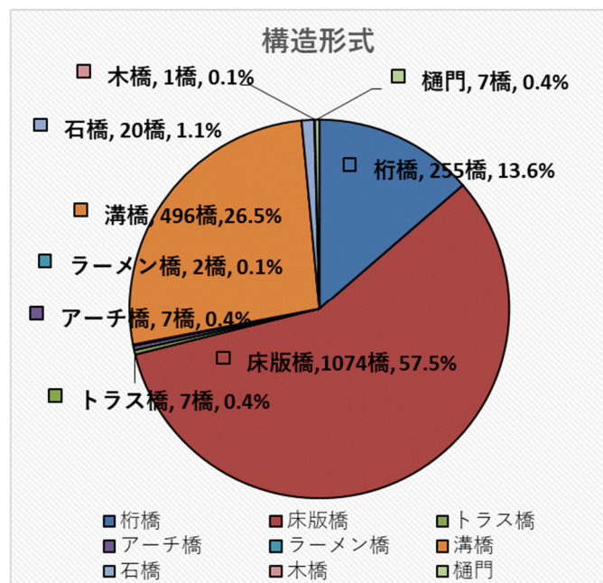
図 1.1.6 構造形式毎の橋梁数
