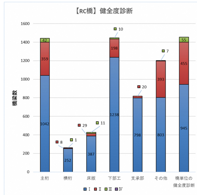
図 1.2.2 RC 橋 健全度診断
