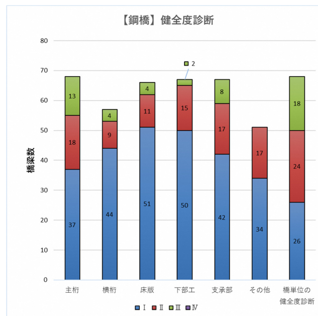
図 1.2.4 鋼橋 健全度診断
