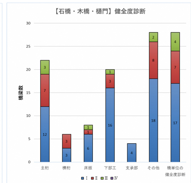
図 1.2.5 石橋・木橋 健全度診断
