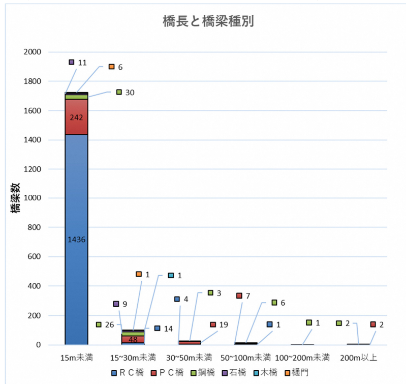
図 1.1.8 橋長と橋梁種別
