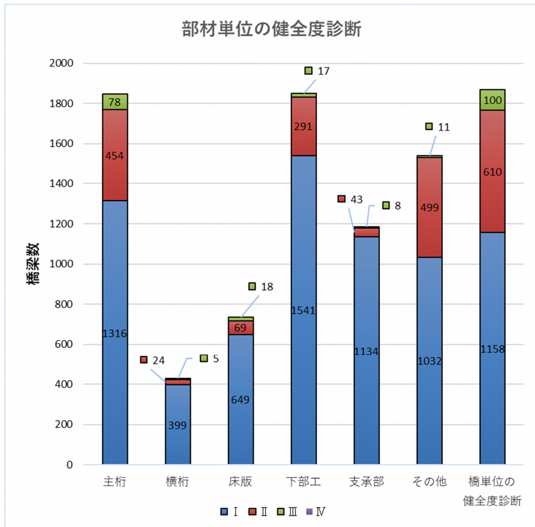
図 1.2.1 部材単位の健全度診断
