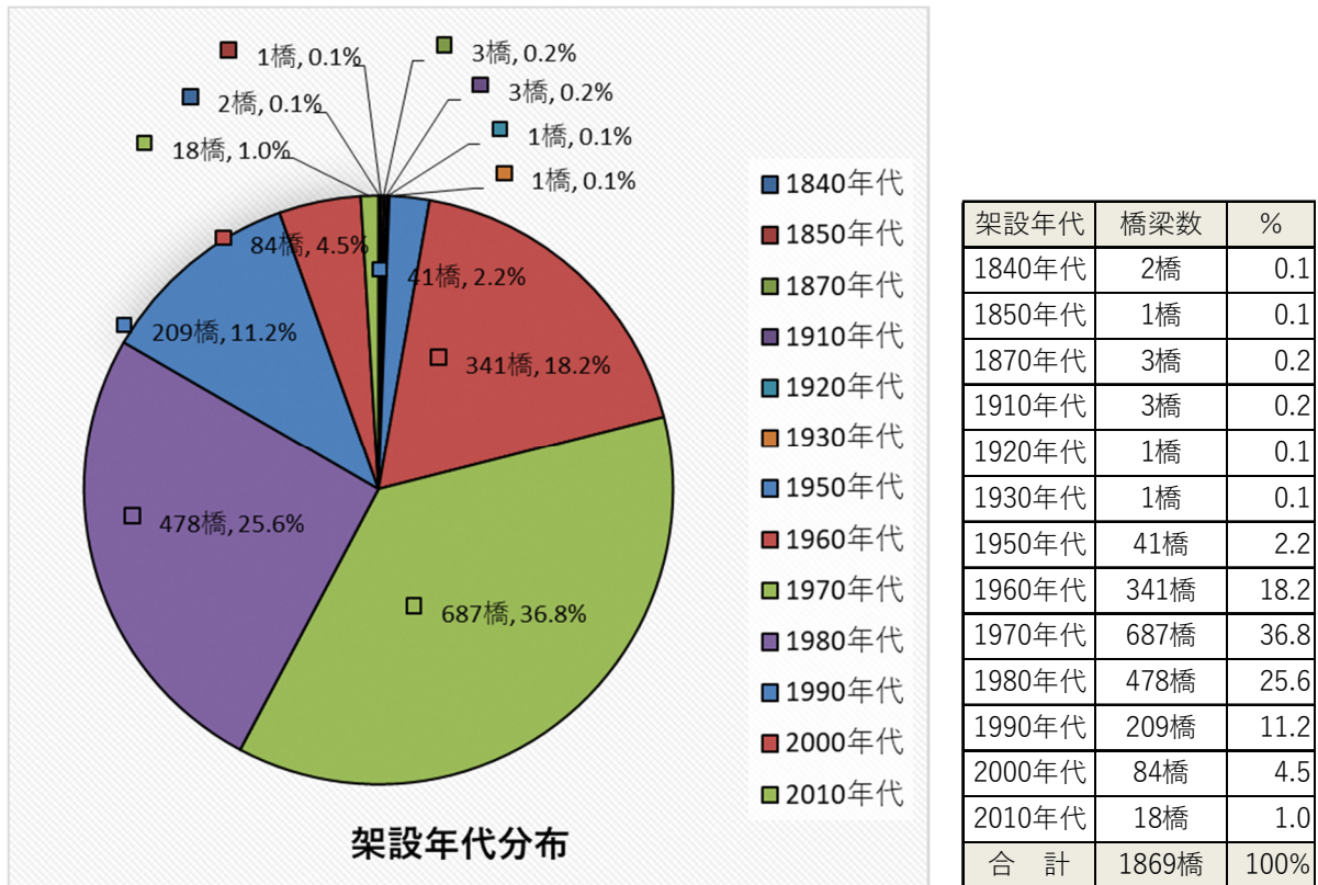
図 1.1.3. 架設年代の分布
