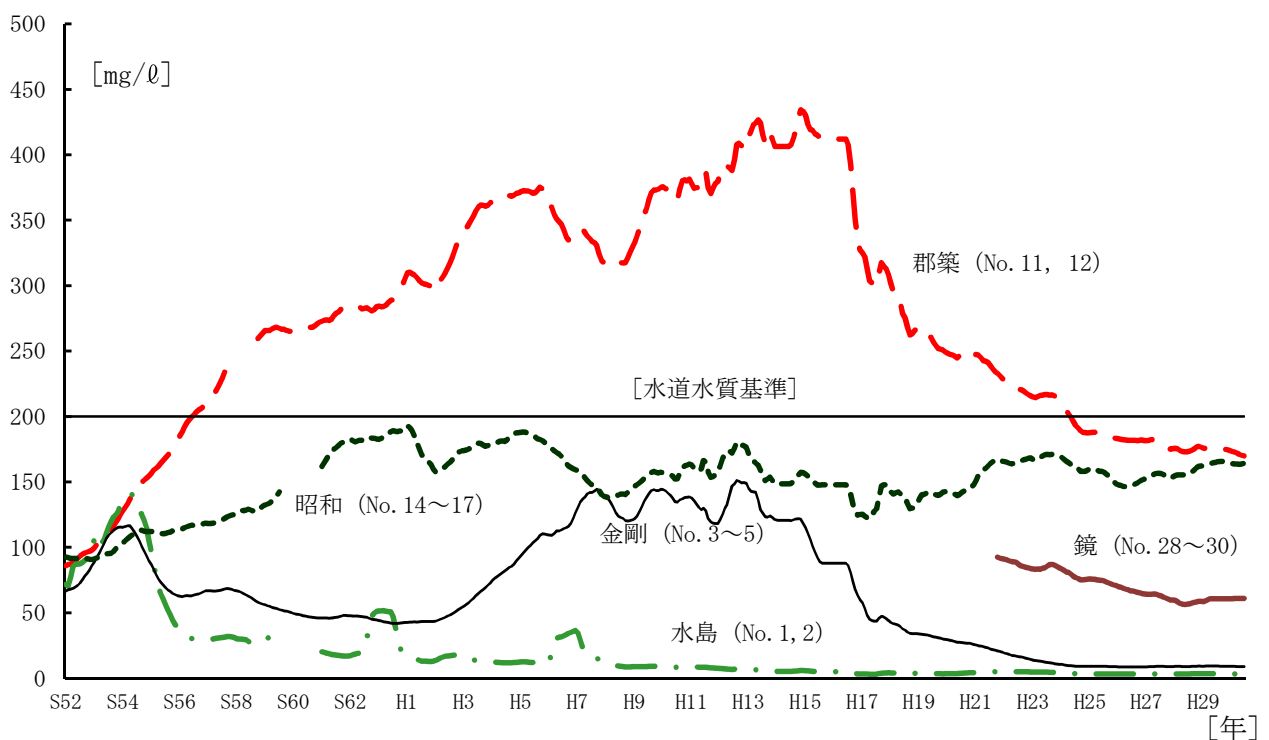
図-9 地域別塩化物イオン濃度の幾何平均の修正移動平均値の推移
