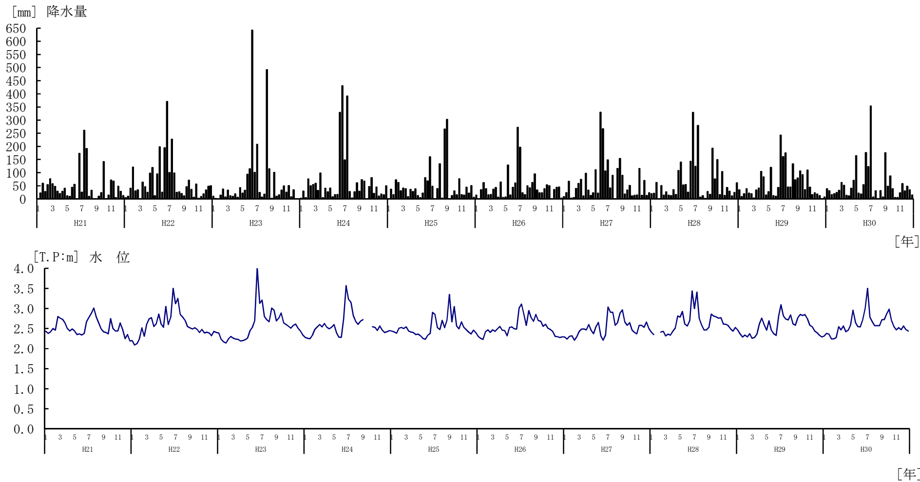
図-4 浅井戸（八代清流高校）の旬平均水位と旬降水量
